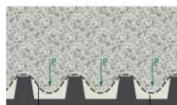
Aiguilleté Noyau incompressible de drainage Cavités drainantes
