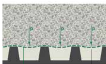
Typar® SF Noyau incompressible de drainage Cavités drainantes
