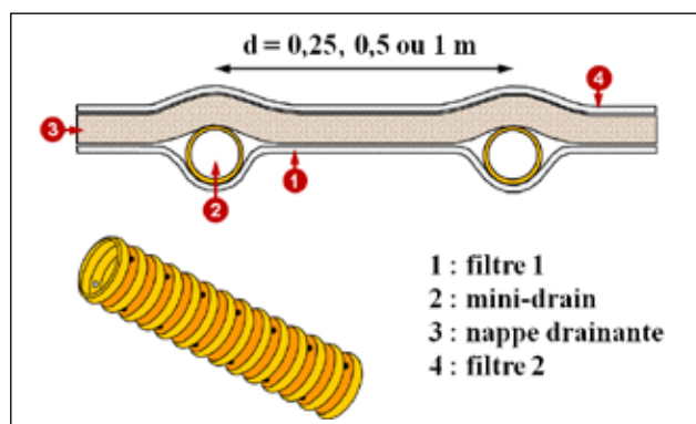
Photo A1 & Figure A1 : les géocomposites de la gamme SOMETUBE 850 FTF D20
