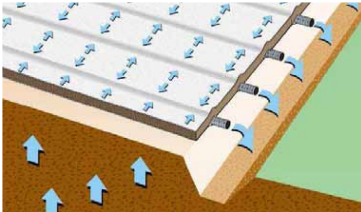
Figure 3 : Les écoulements dans les géocomposites de la gamme SOMTUBE 850 FTF D20
