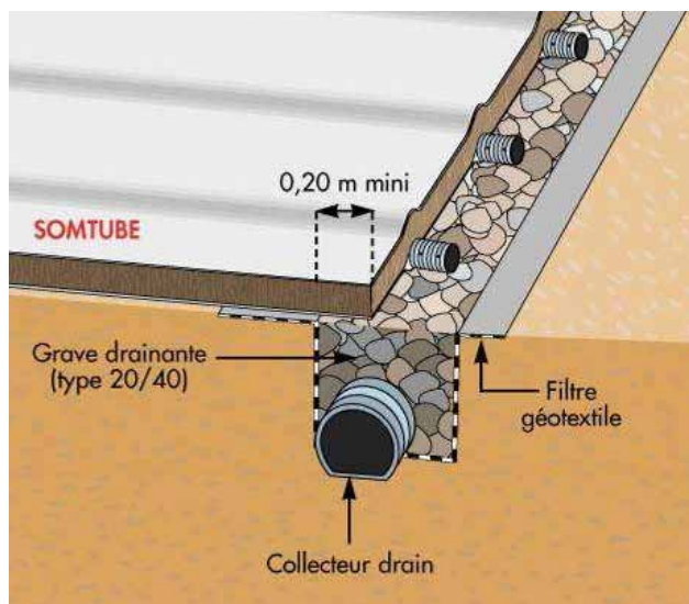
Figure A5 : Raccordement à la tranchée
