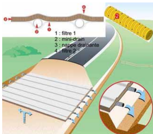
Figure A2 : Principe de déroulement des géocomposites de la gamme SOMTUBE 850 FTF D20
