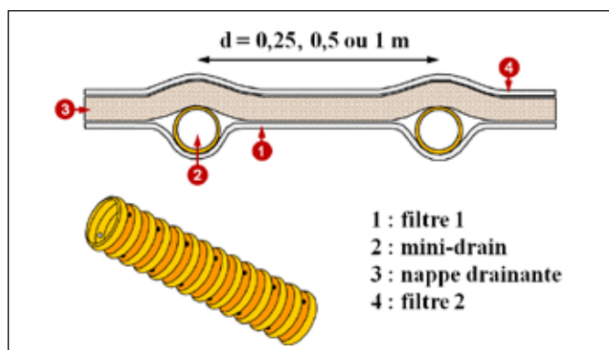
Figure 1 : Structure des géocomposites de la gamme SOMTUBE 850 FTF D20
