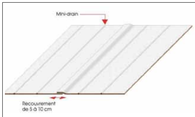
Figure A4 et photo A7 : Traitement des joints longitudinaux (côte à côte)
